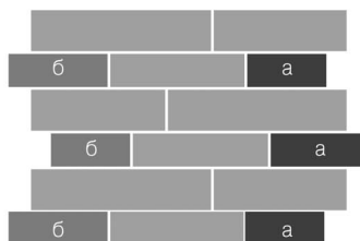
2 Вид плитки при укладке
